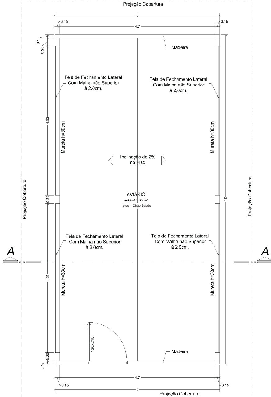
PLANTA BAIXA Área=50.00 m 2 Sem Escala
