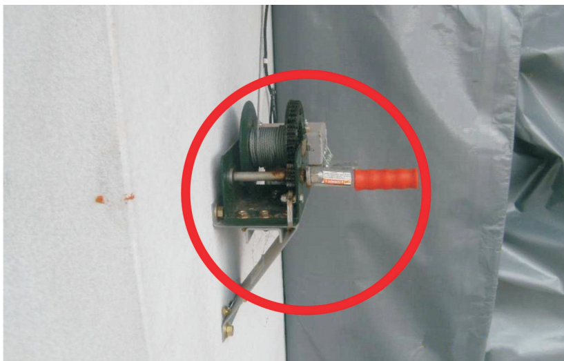
Fig. 4. Catraca para movimentação da cortina lateral.
